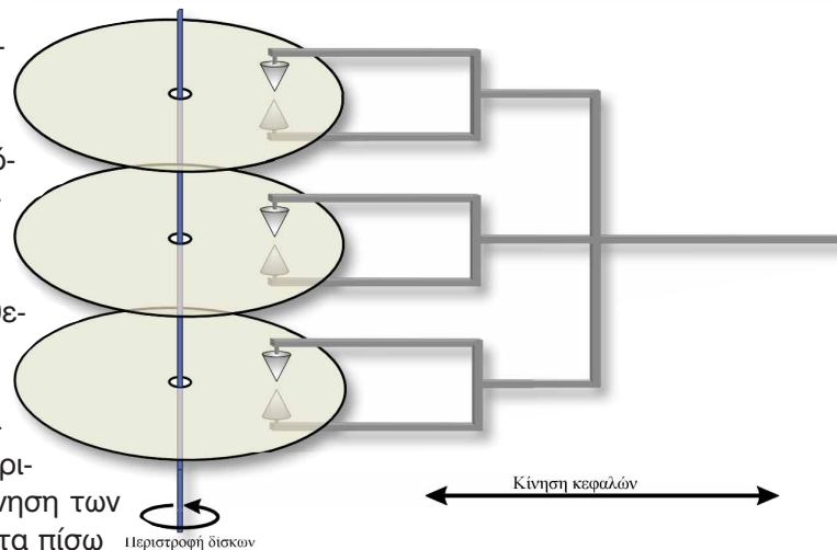
Σχήμα 3.4 Σκληρός δίσκος
